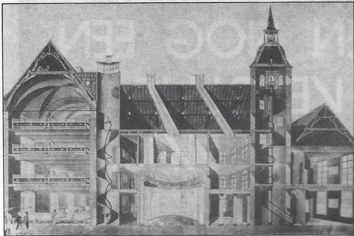
Lengtedoorsnede van de katoenspinnerij van L. Bauwens (1808) foto ACL/B149447
