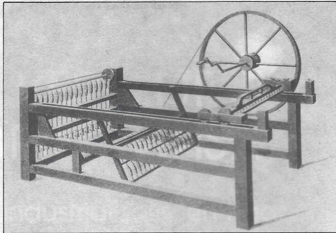
Spinning Jenny foto Provinciaal Tekstielmuseum Vrieselhof
